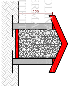
SEZIONE A-A
