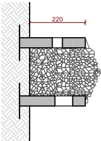
SEZIONE A-A
