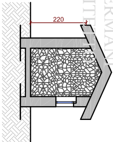
SEZIONE A-A
